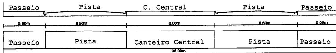
Detalhe - Seção Tipo da Av. das Figueiras Trecho 01 - Largura de 35,00m
