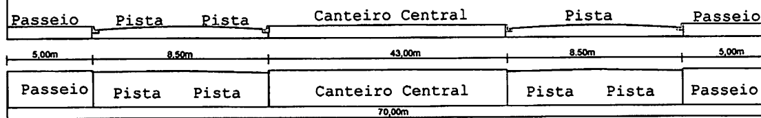
Detalhe - Seção Tipo da Av. das Figueiras Trecho 03 - Largura de 70,00m
