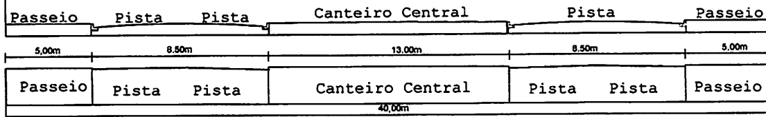
Detalhe - Seção Tipo da Av. das Figueiras Trechos 03 e 05 - Largura de 40,00m
