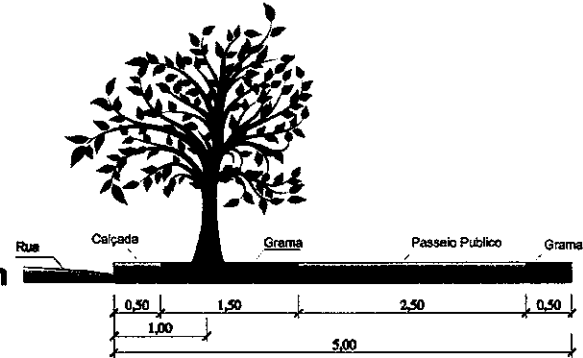
Calçada Largura 5,00m
