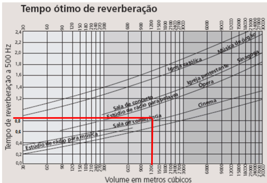
Figura 4: Ábaco do Tempo de Reverberação para 500Hz – Auditório 01
